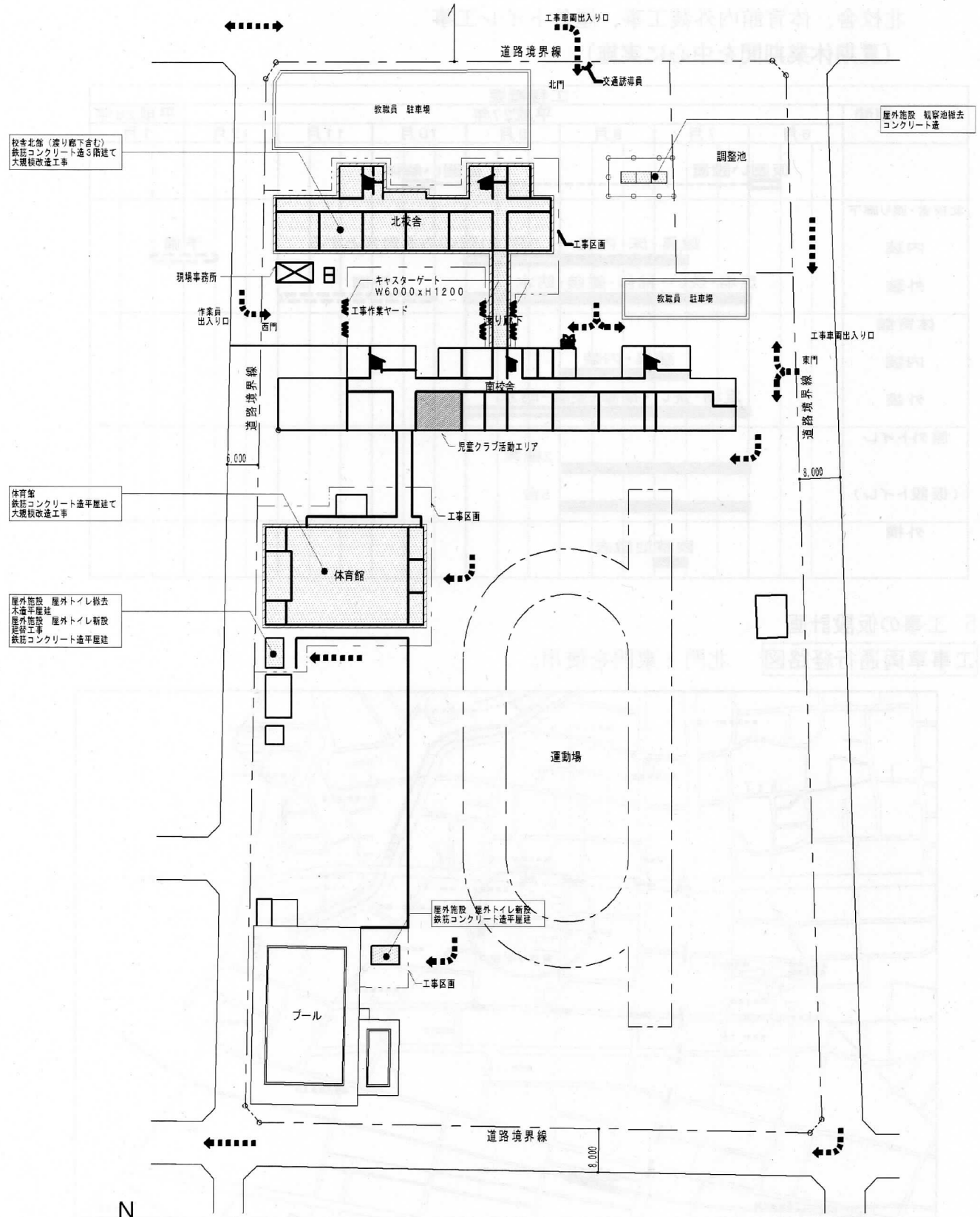
配置図
